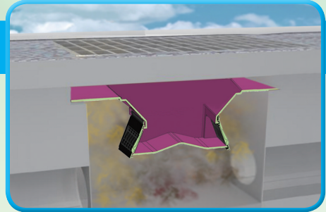
차단판 닫힘 ➡ 악취 차단
