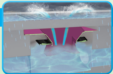
차단판 열림 ➡ 하수 배출
